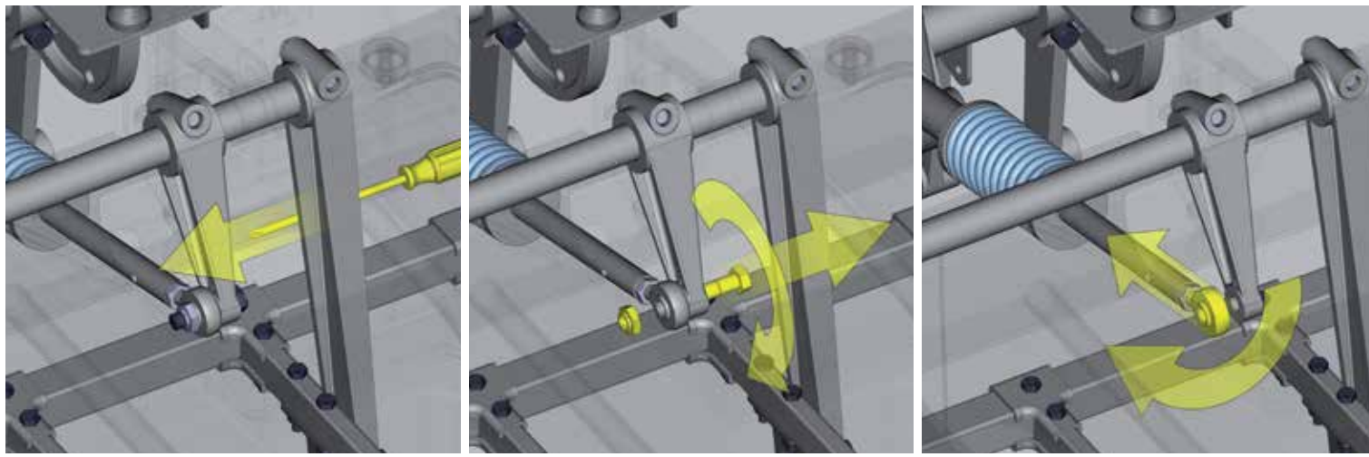
Demos des EDGE Video-Schulungsinstruments, die die Einstellung der Shuttlestange am Pinspotter zeigen
